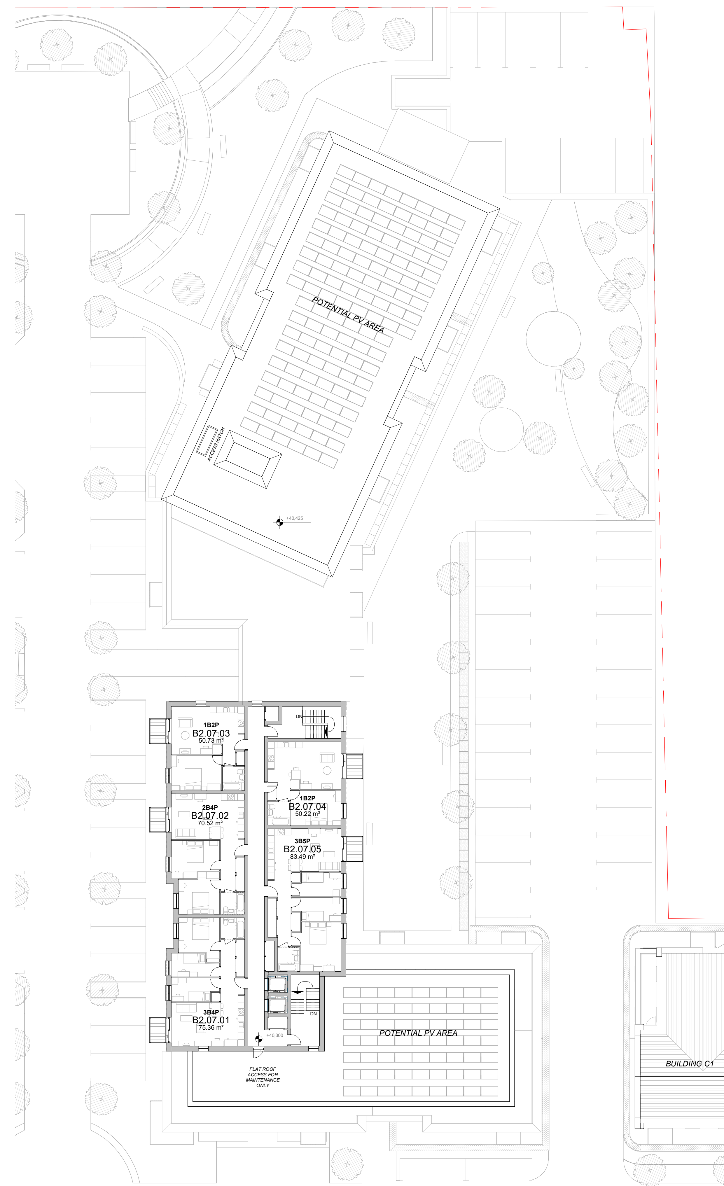
2 Level 7 +34.300 AOD 1:200
