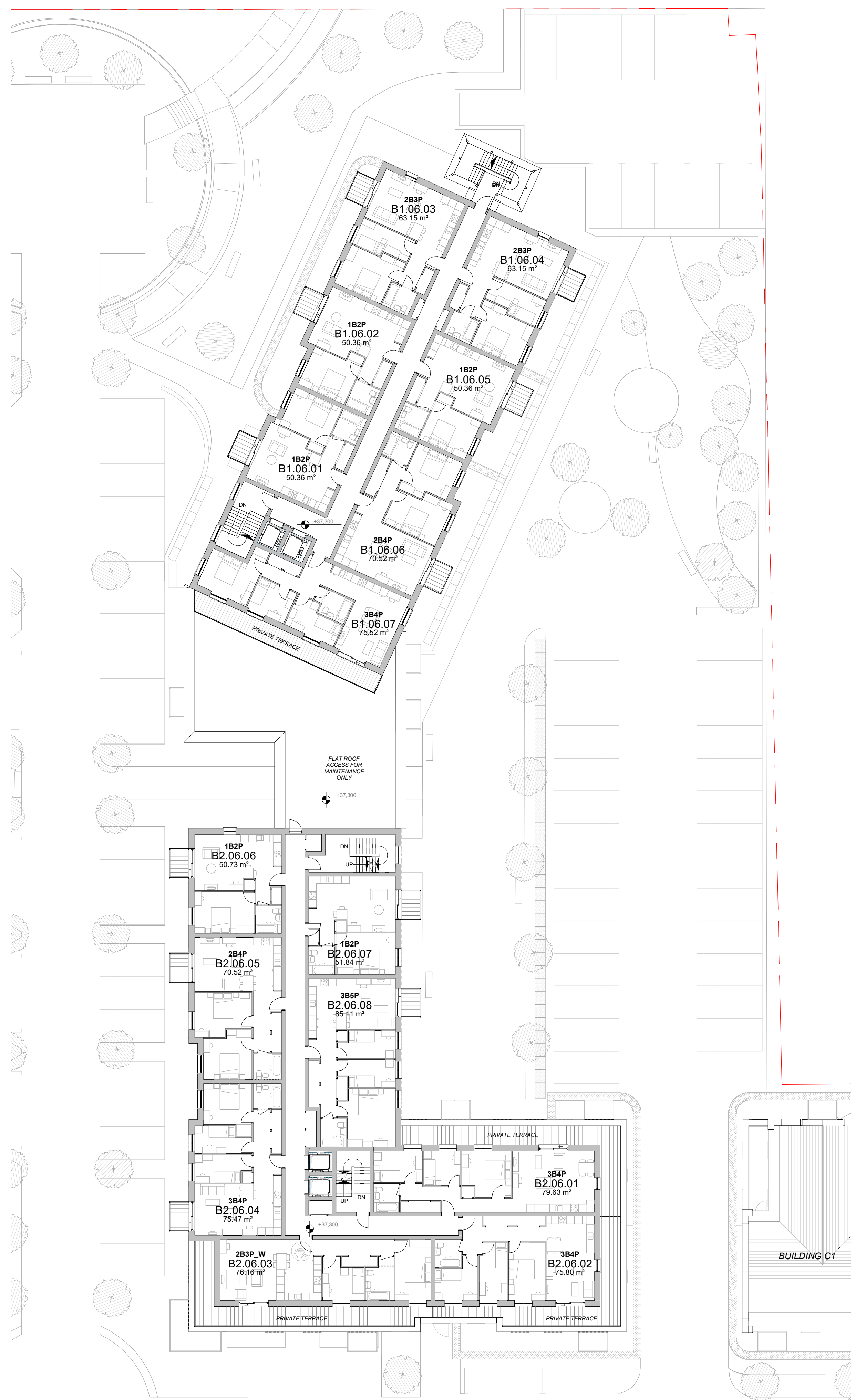
1 Level 6 +37.300 AOD 1:200
